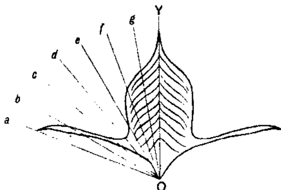
Fig. 412. Cleodora cuspidata .
