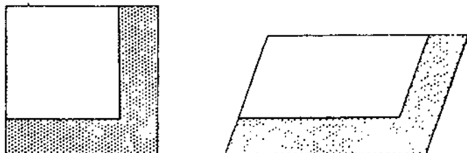
Fig. 354. Gnomonic figures.
